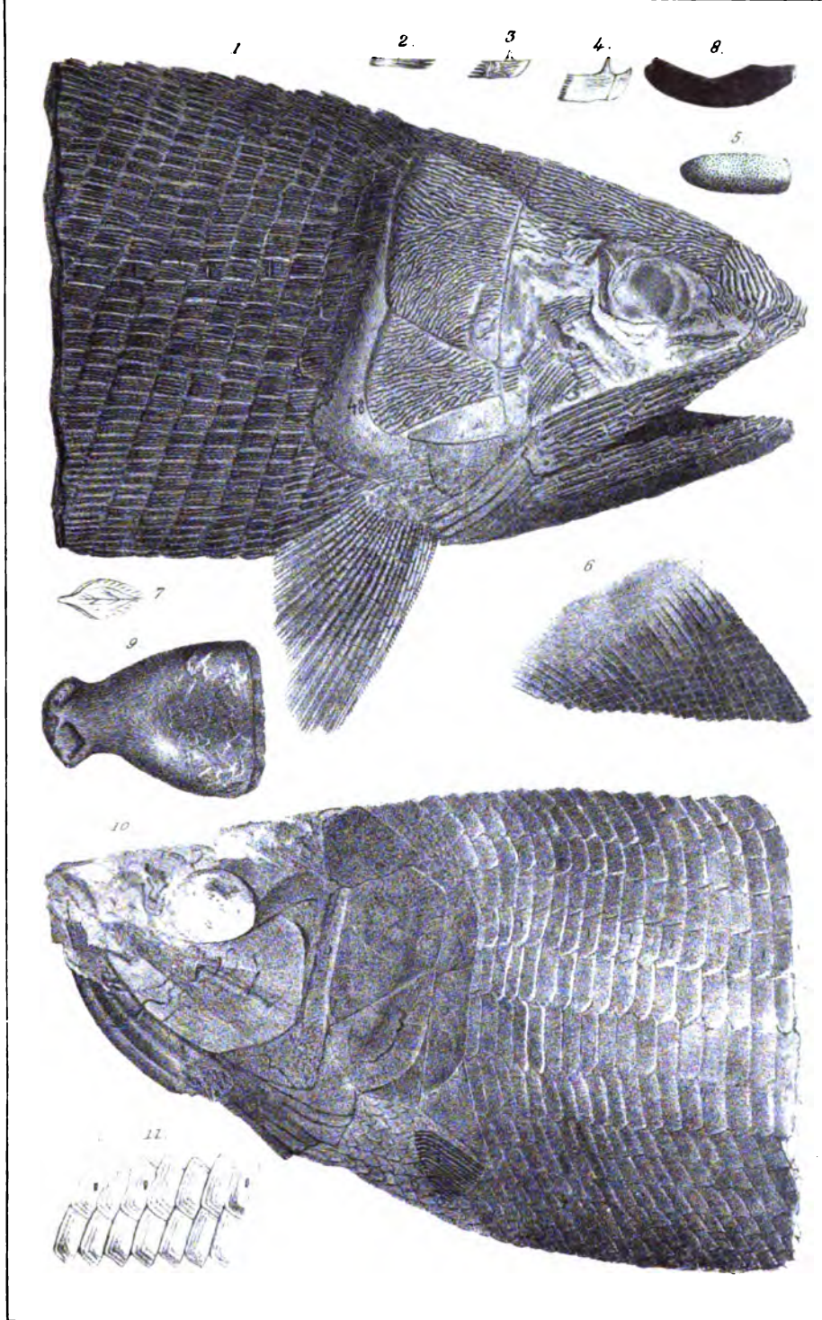
Guenstede, Jura.
